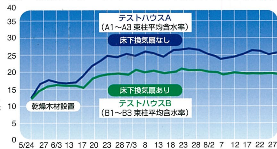
含水率 (%) 《当社テストハウスにおける床下束柱木材含水率比較》
